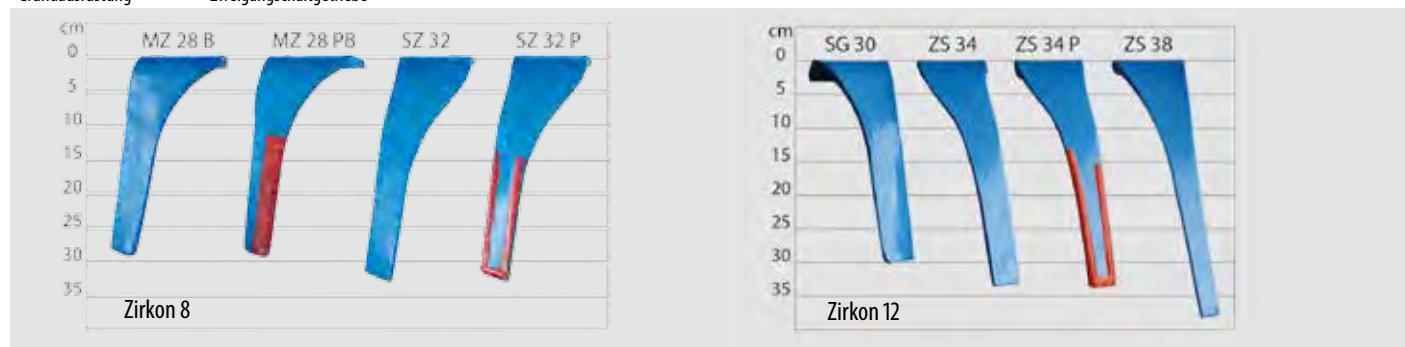
Kreiseleggen-Zinken für verschiedene Einsatzbereiche, auf Wunsch auch mit Aufpanzerung für höchste Standzeiten (im Bild rot markiert)
